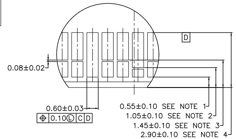
DETAIL AB SCALE 2:1
