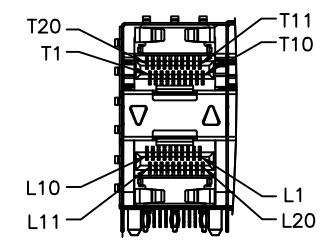
DETAIL A 1:1
