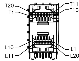
DETAIL A 1:1
