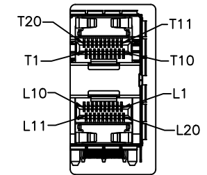
DETAIL A 1:1
