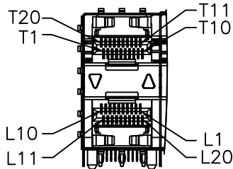
DETAIL A 1:1
