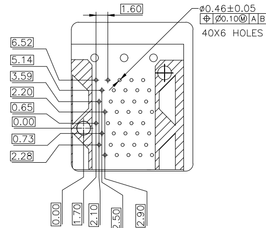
DETAIL H 2:1
