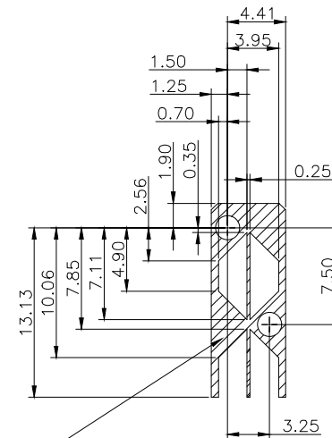
DETAIL H 2:1
