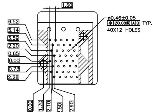
DETAIL H 2:1
