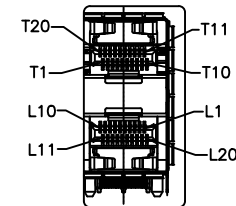
DETAIL A 1:1
