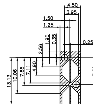
DETAIL H 2:1
