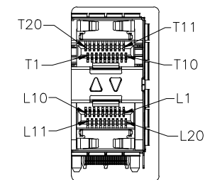
DETAIL A 1:1
