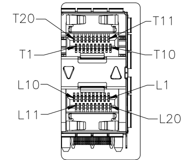
DETAIL A 1:1
