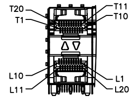
DETAIL A 1:1
