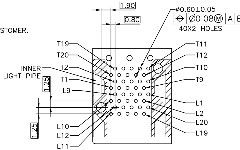
DETAIL H 2:1
