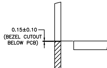
DETAIL K 2:1
