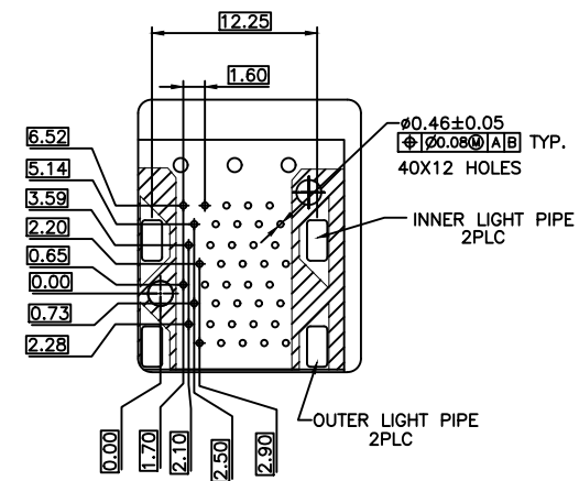
DETAIL H 2:1
